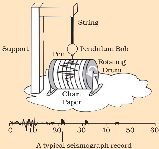
Fig. 12.13 : A seismograph
