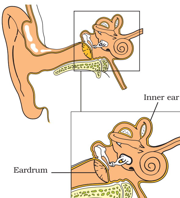
Fig. 10.16 : Human ear
